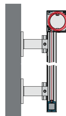
Micro 860 (zip) Monteret med afstandstykker
