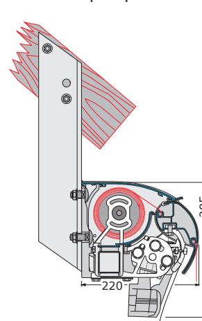
Monteret på spærside
