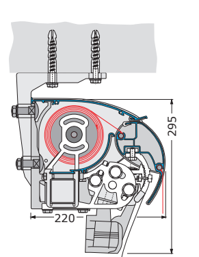
Monteret på spærside
