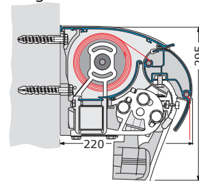
Monteret under udhæng
