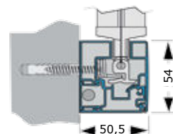
Dimensioner på sideskinne
